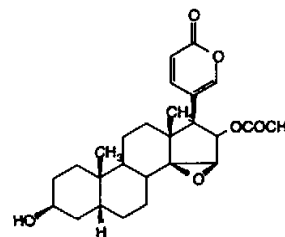
Cinobufagin
